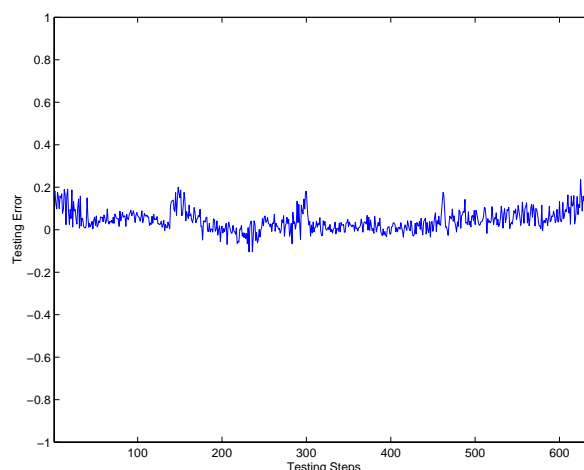
Fig. 10. Testing Error
